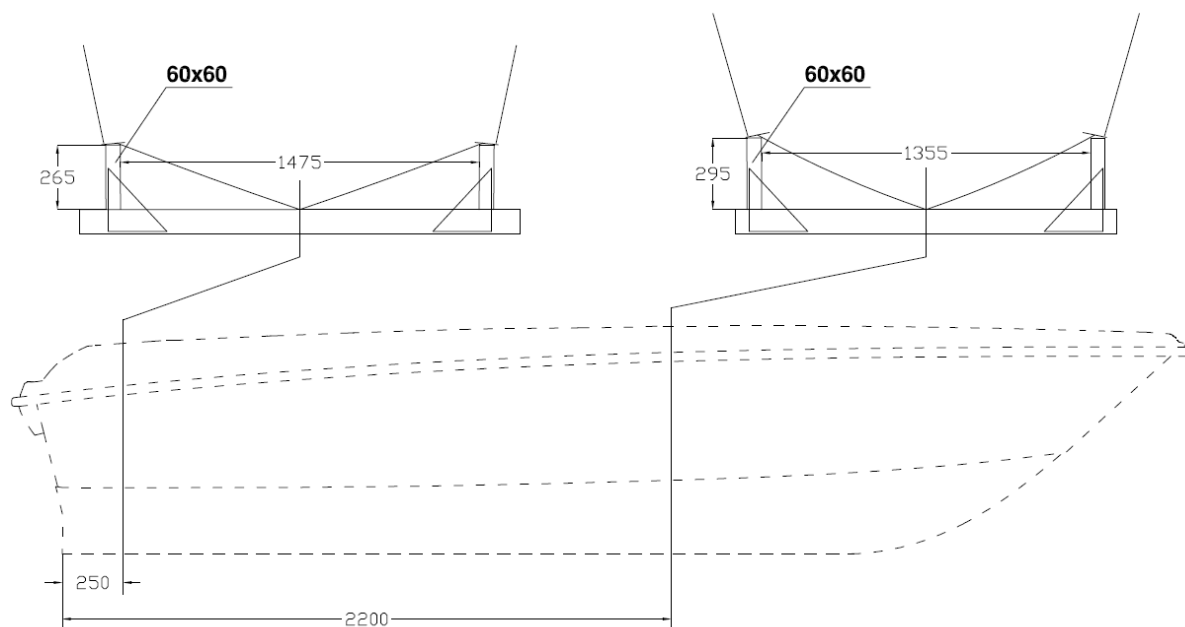
Bild: Båtbockarnas dimensioner.
