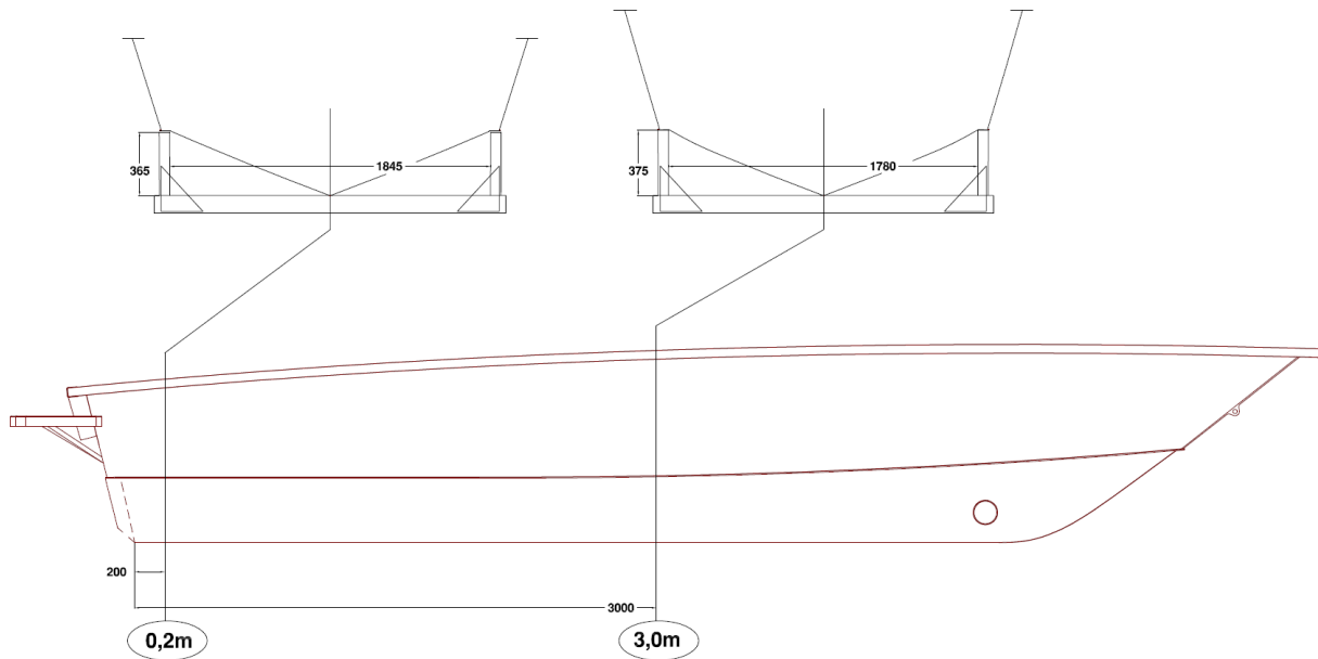
Talvisäilytyspukkien mitat
